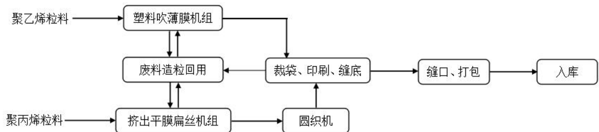
图 1 生产工艺流程
