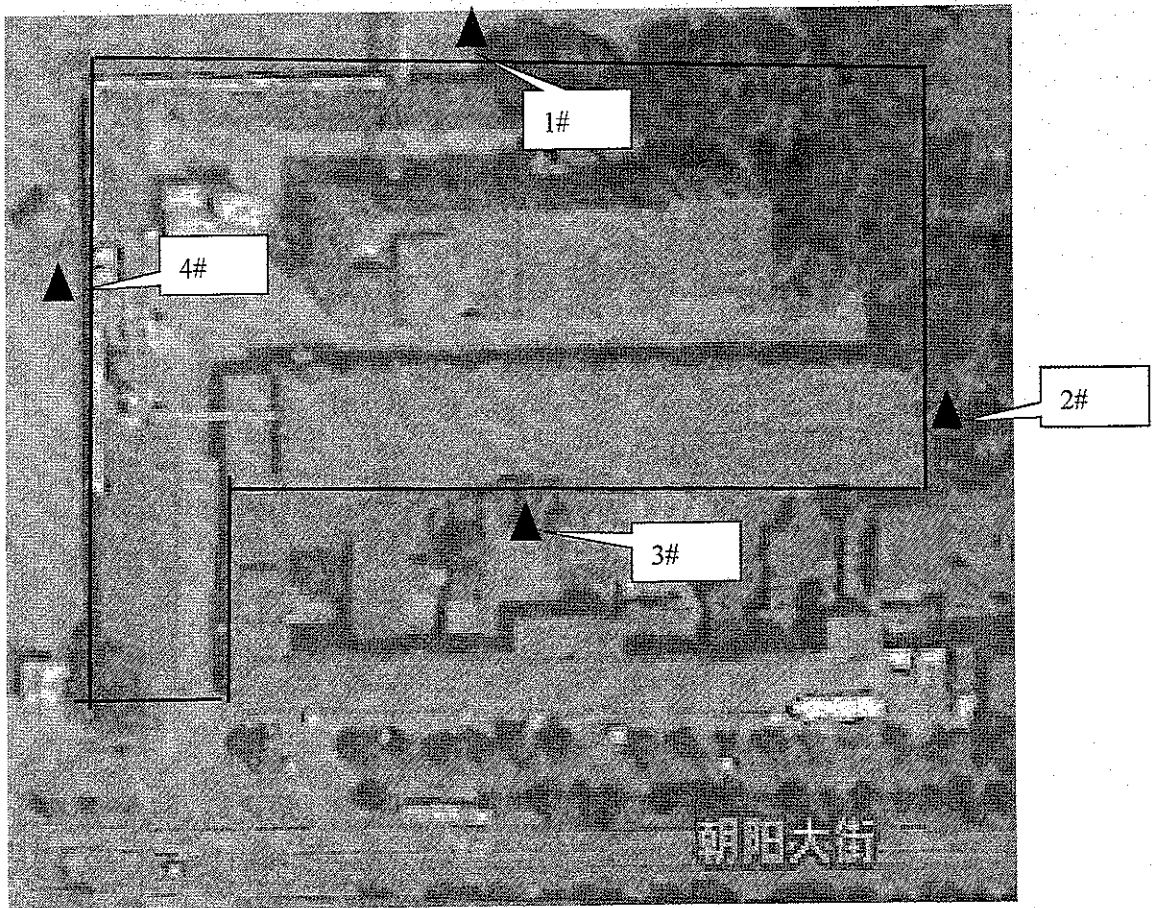
附图 1: 陕西渭河塑业有限责任公司厂界噪声点位示意图
